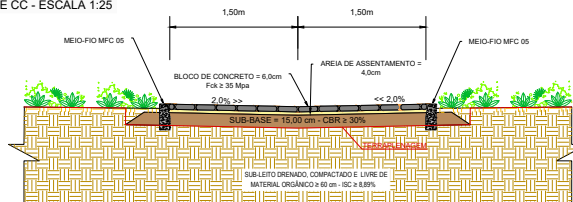
CORTE CC - ESCALA 1:25
