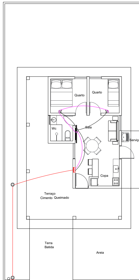
Planta Baixa - Layout Normal
