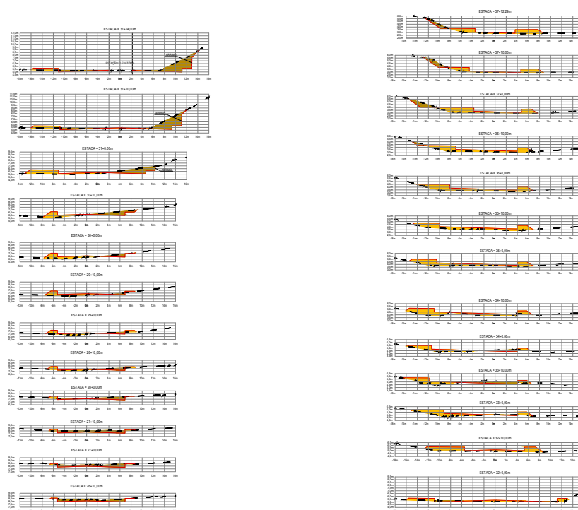
SEÇÕES TRANSVERSAIS DO EIXO 01
